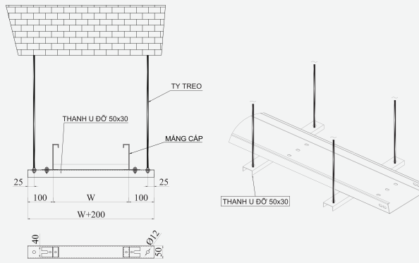
U ĐỒ MÁNG Trapeze Hanger
