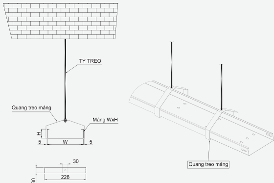
QUANG TREO MÁNG Hanger Brackets
