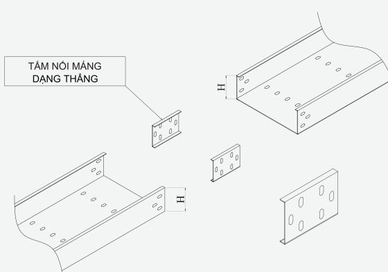
NỐI MÁNG DẠNG THẰNG Splice Plates
