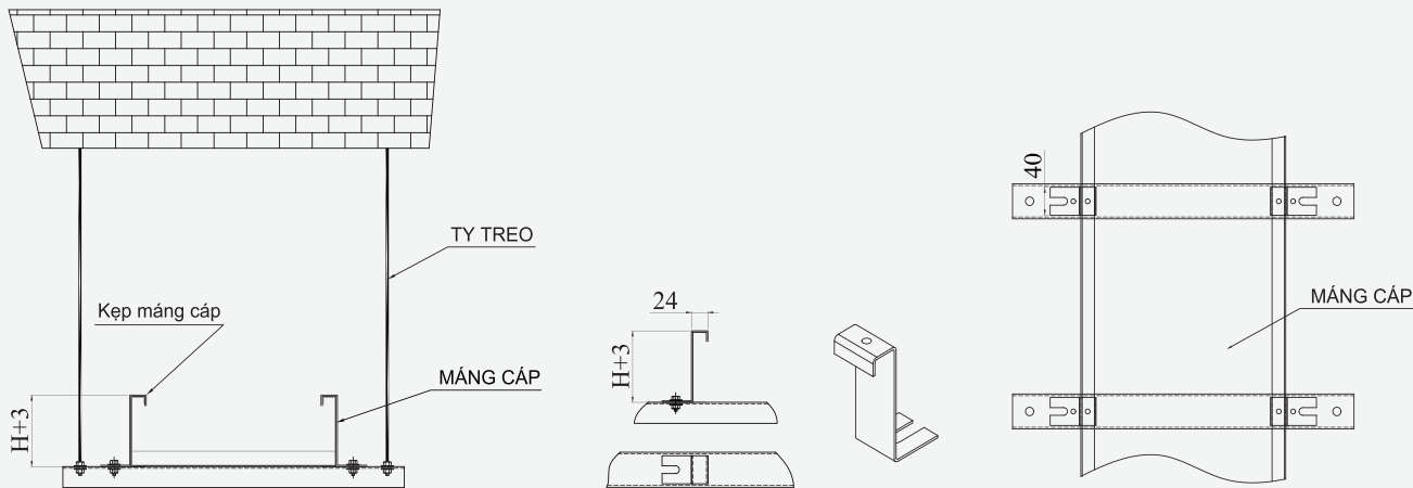
KẸP MÁNG CÁP Clamp
