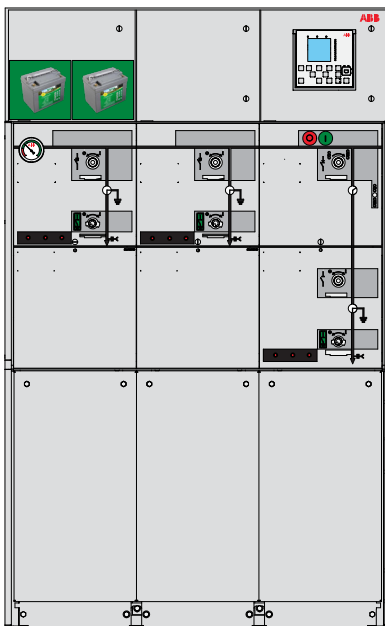
300mm LVC
